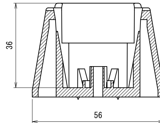
断面 A-A
